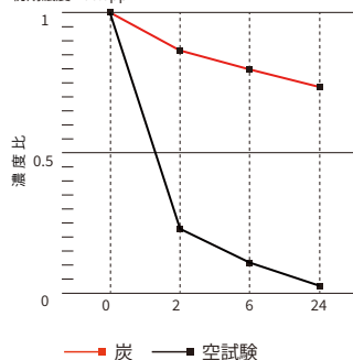
アンモニアの減少率
