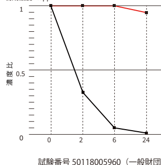
硫化水素の減少率
